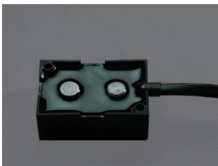
Unterseite mit zwei Edelstahlelektroden
