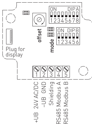
Схема подключения
