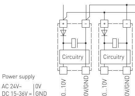
Схема соединения
