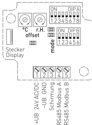
Schaltbild
